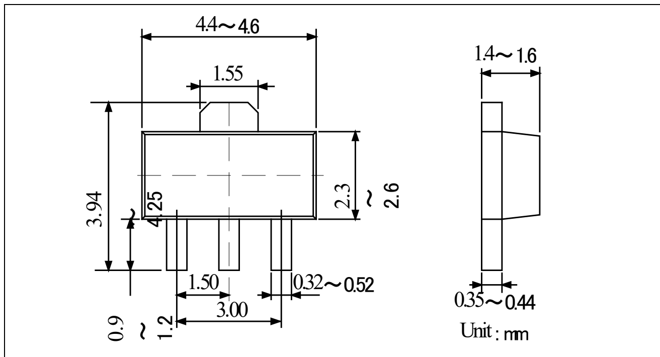
SOT89-3
