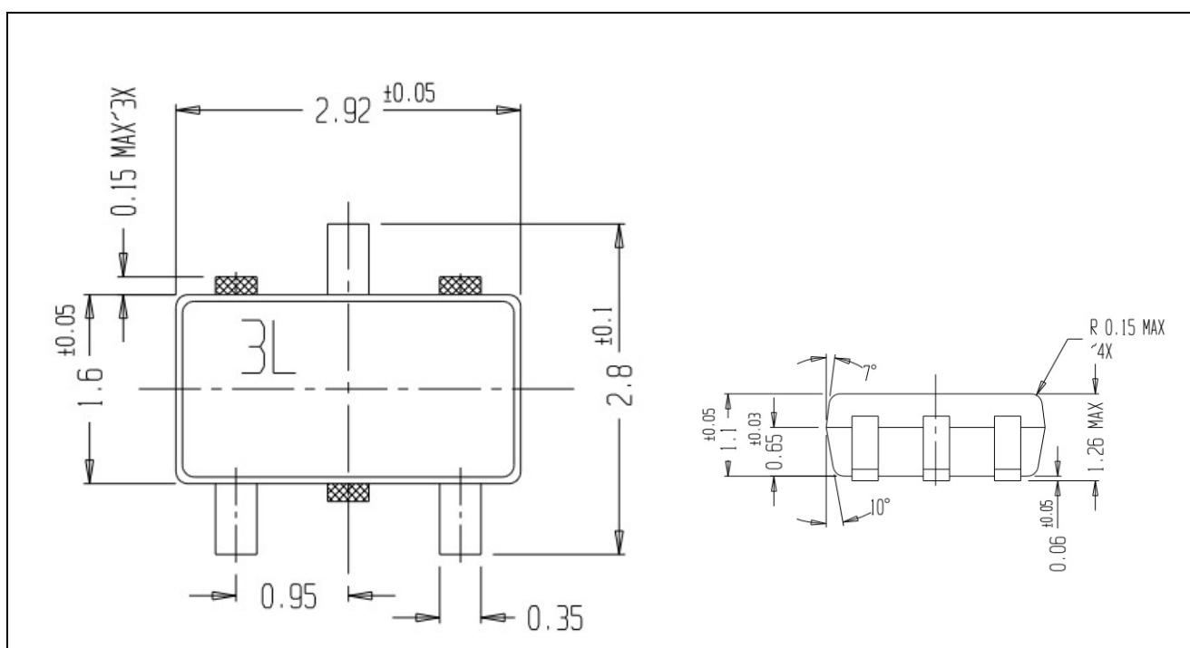
SOT23-3L
